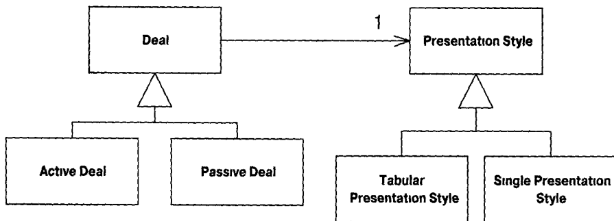
Рис. 12.5. Теперь иерархии разделены
