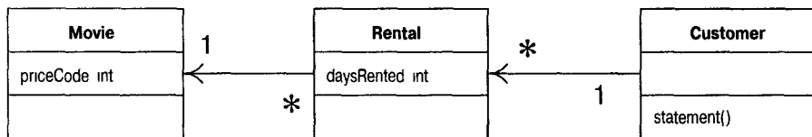
Рис. 1.1. Диаграмма классов для исходной программы. Нотация соответствует унифицированному языку моделирования [Fowler, UML]
