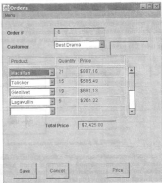
Рис. 12.7. Интерфейс пользователя в начальной программе
