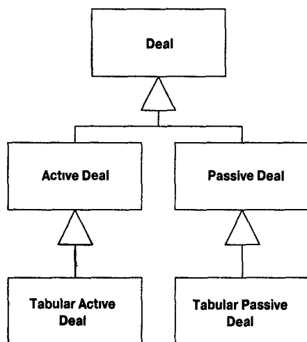
Рис. 12.1. Запутанная иерархия
