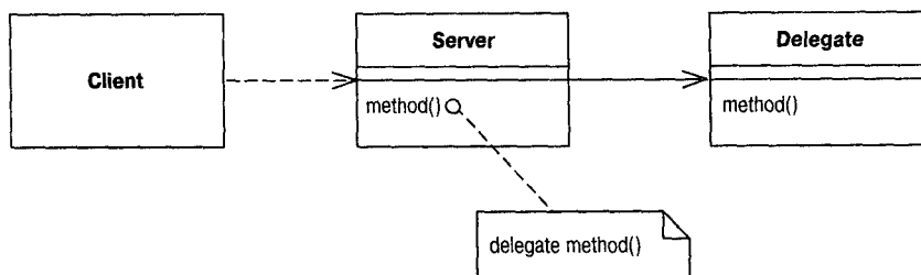
Рис. 7.1. Простое делегирование
