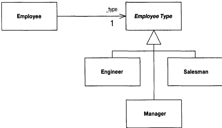
Рис. 9.1. Структура наследования
